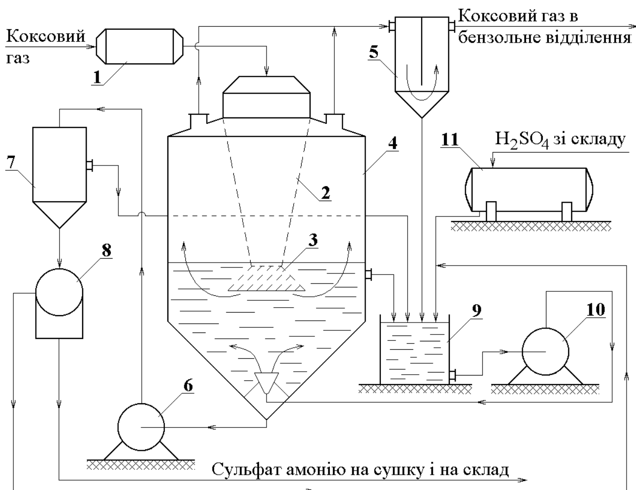
Рис. 2.1. Технологічна схема сульфатної дільниці коксохімічного заводу:
