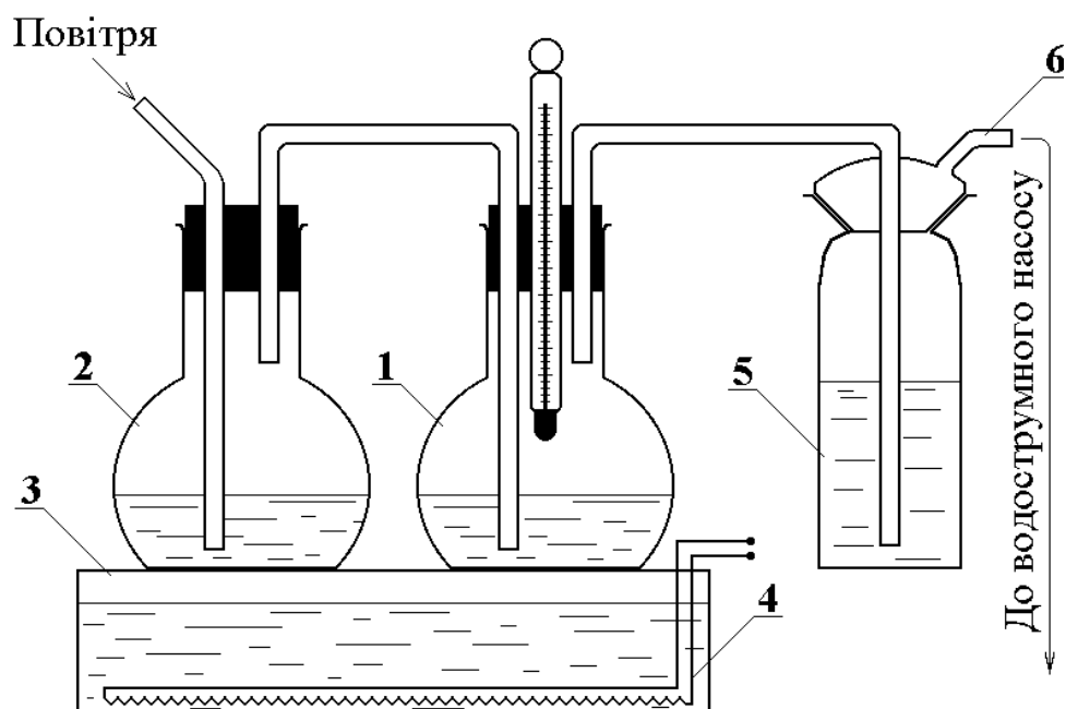
Рис. 4.1. Схема лабораторної установки для одержання амоній сульфату:
