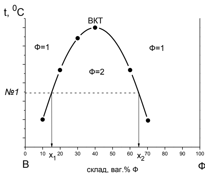
Рис. 3.1 – Діаграма взаємної розчинності двох обмежено розчинних рідин (діаграма ліквіації)
