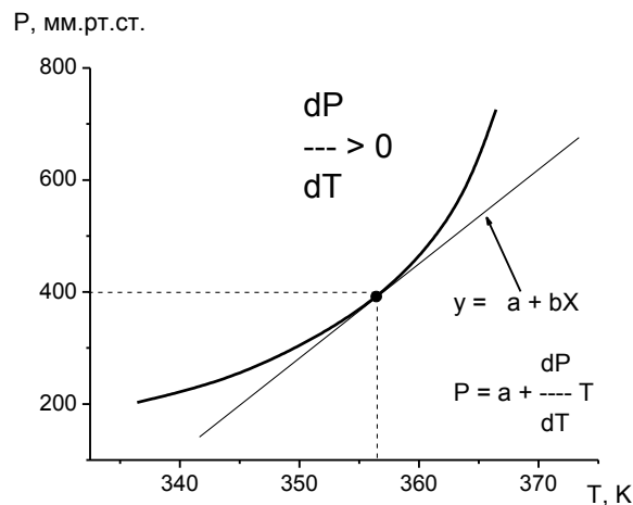
Рис. 1.1 – Залежність тиску насиченої пари рідини від температури або температури її кипіння від зовнішнього тиску
