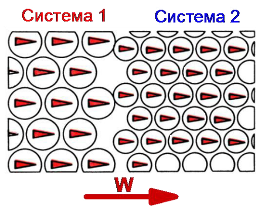
Рис. 1.2. Система 2 усваивает упорядоченность (когерентность) движения частиц Системы 1. Система 1 совершает работу над Системой 2
