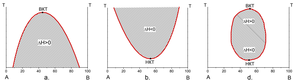
Рис.4.16 Типичные системы с ограниченной взаимной растворимостью жидкостей: а – система с верхней критической температурой растворения; б – система с нижней критической температурой растворения; д – система с верхней и нижней критической температурой растворения
