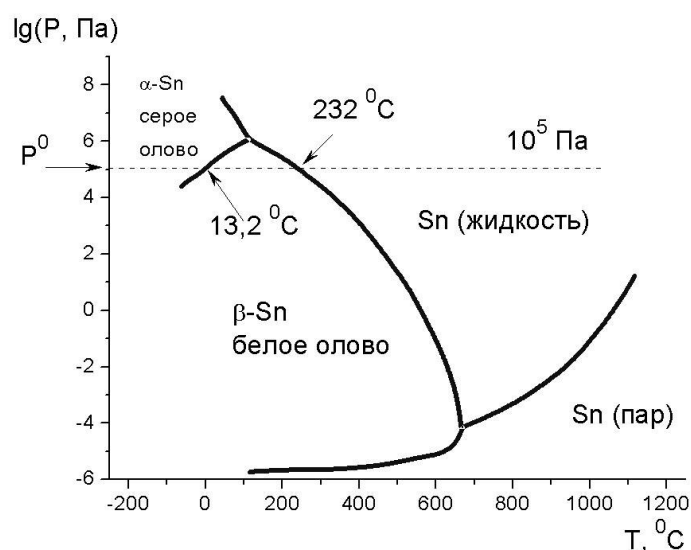
Рис.3.12 Диаграмма состояния олова (металлическое олово имеет температуру плавления 231,84 ^\circ\text{C} и нормальную температуру кипения 2362 ^\circ\text{C} , его пары окрашены в голубой или серо-голубой цвет).
